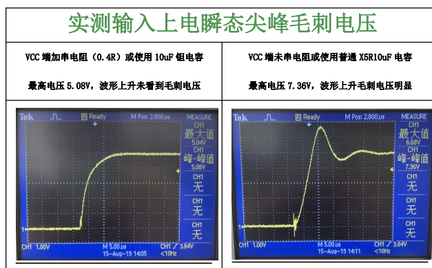
图3：5V上电波形图
