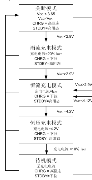
图 1: 一个典型充电循环的状态图
