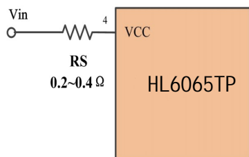
图2：一种尽量增大热调节模式充电电流的电路
