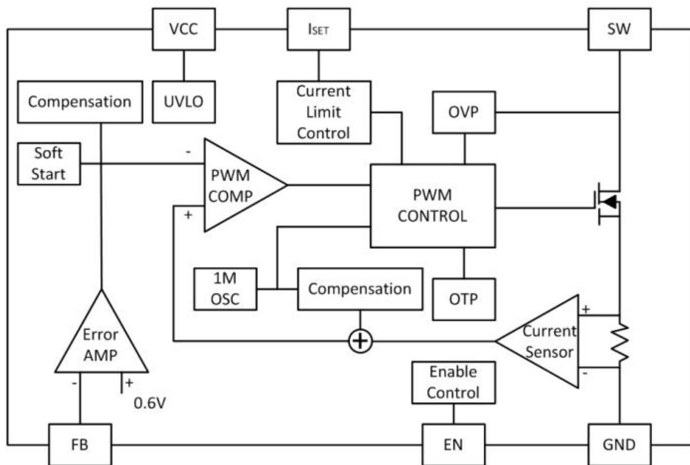
结构框图
